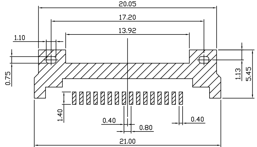
P.C.B LAYOUT
