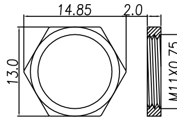
NUT
